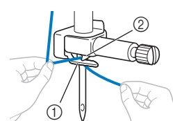
① Guide-fil de la barre de l'aiguille ② Taquet
